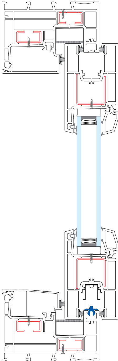
A - A
